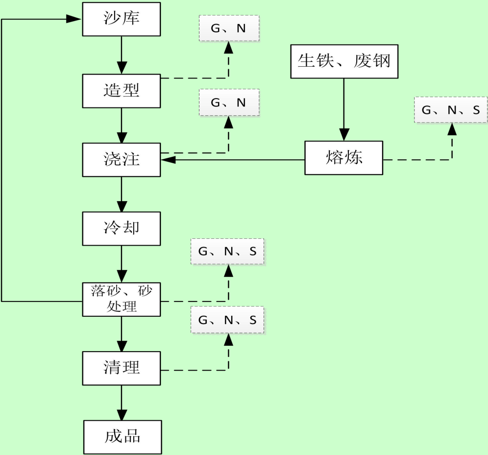
图 1 技改项目运营期工艺流程及产污环节示意图
