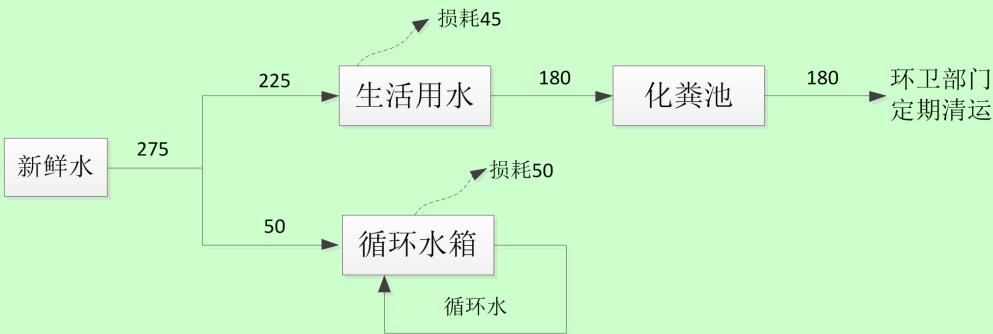
图 2.2-2 项目水量平衡图 单位：m³/a
