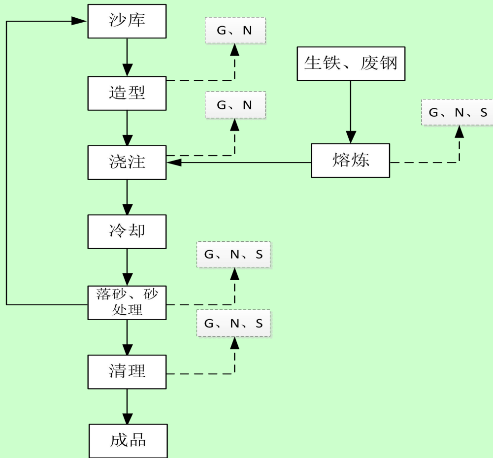
图 2.3-2 铸造生产工艺及产污环节示意图
