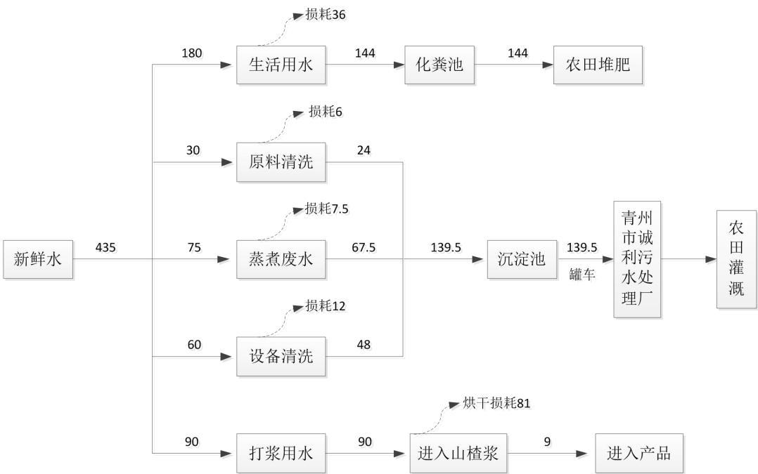
图 2.2-2 项目水量平衡图 单位：m³/a
