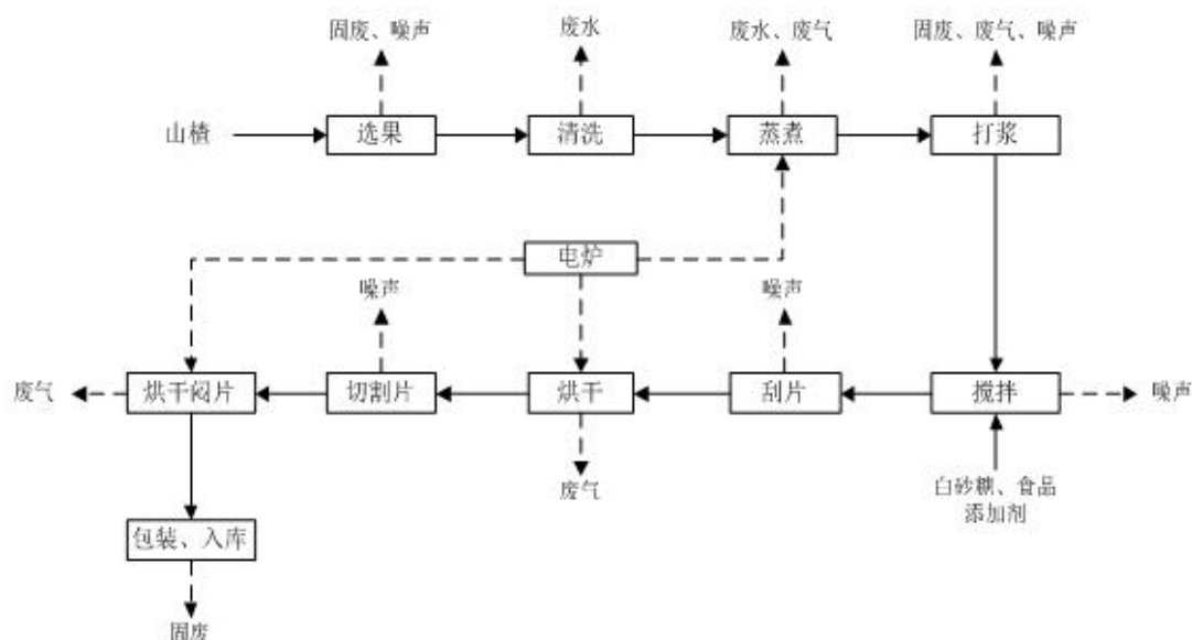
图 1 工艺流程及产污环节示意图
