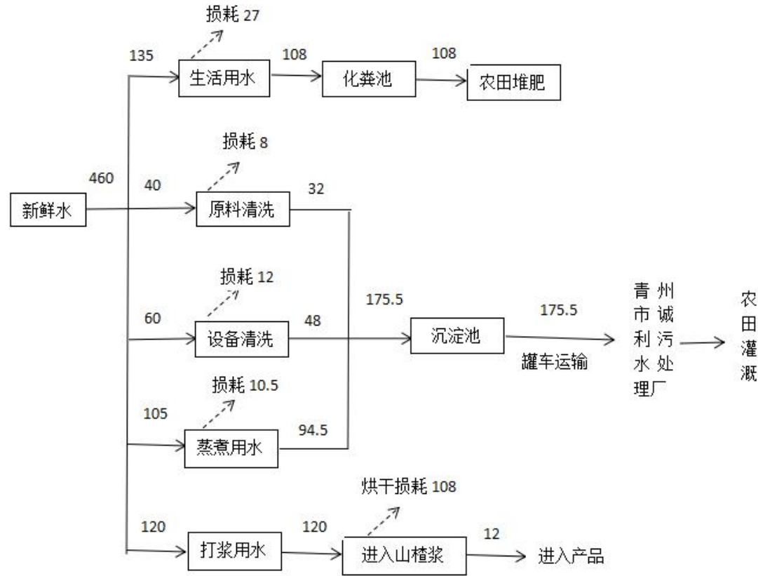
图 2.2-2 项目水量平衡图 单位：m³ /a
