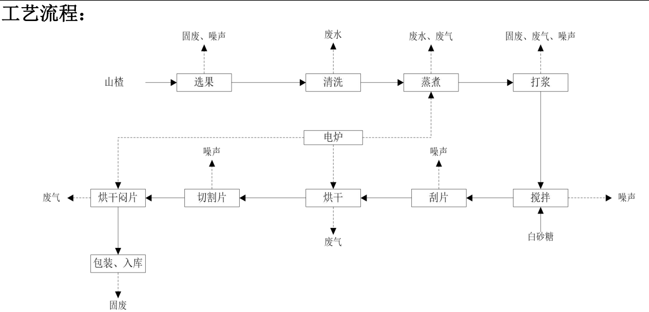
图 1 工艺流程及产污环节示意图
