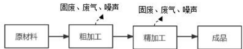
图2.3-1 其他机械配件生产工艺流程及产污环节示意图
