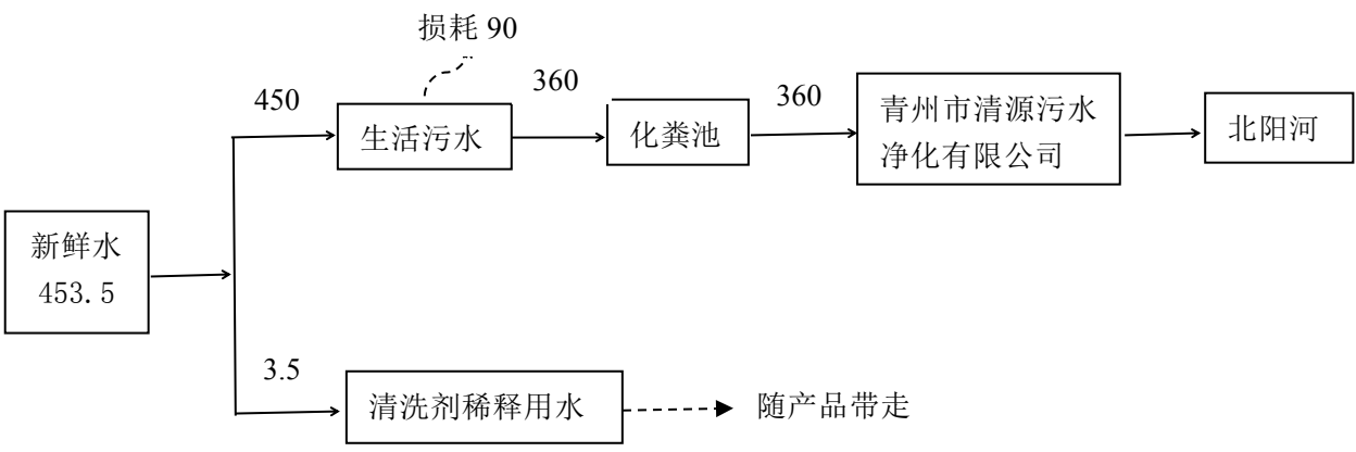
图2.2-1 项目水平衡图 单位: m 3 /a
