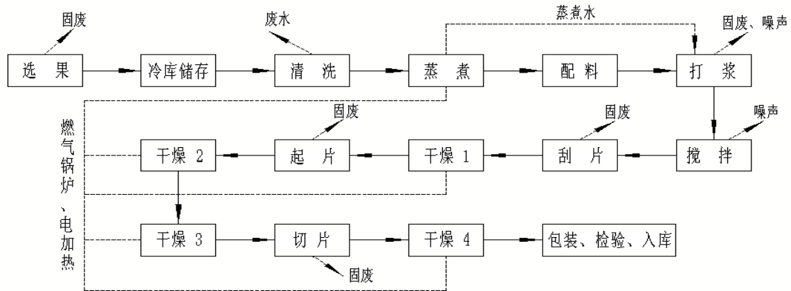
图 2.3-1 工艺流程及产污环节示意图
