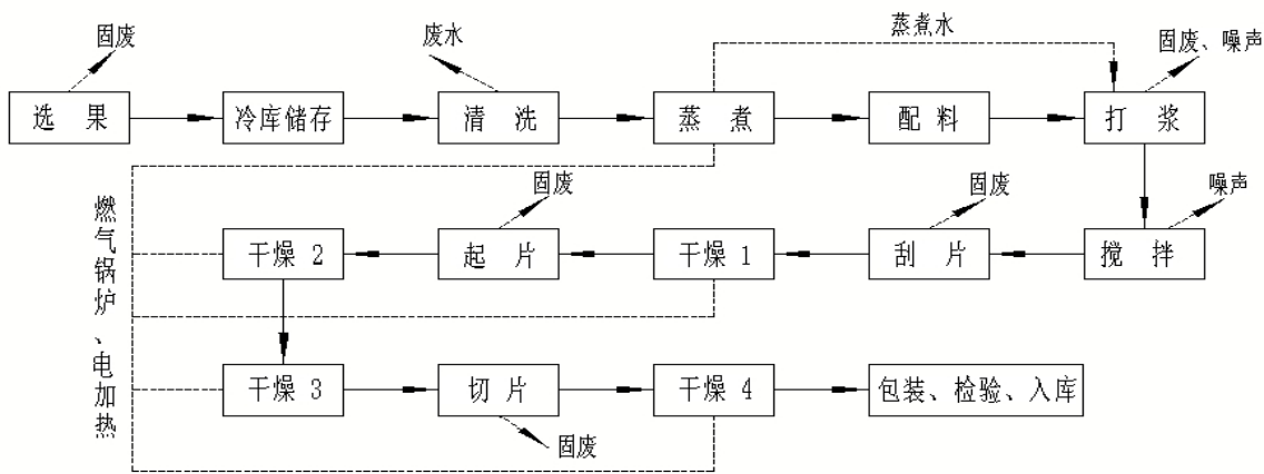
图 1 工艺流程及产污环节示意图
